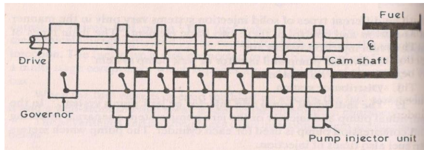
Fig. 19. Unit injector
