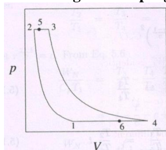
P-V diagram
