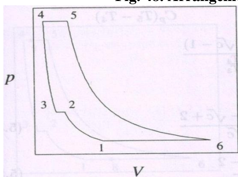
P-V diagram
