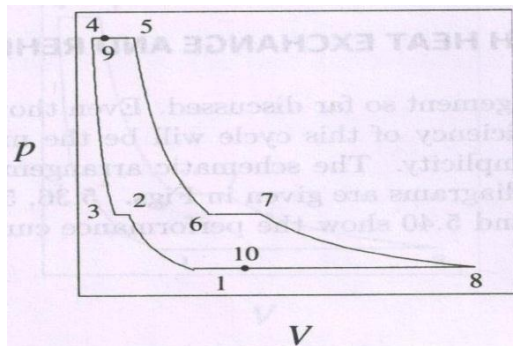
P-V diagram
